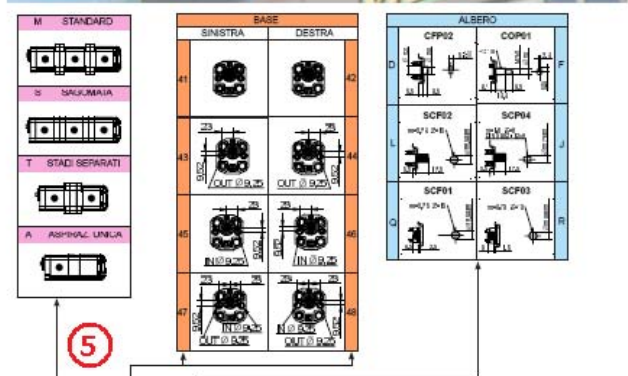
POMPA MULTIPLA XV-1 BASE # 32 Sagomata - TIPO "BH"
